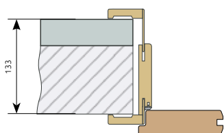
obl. zárubeň B (95-115 mm) síla stěny 133 mm záklopový límec s delším spojovacím perem +18 mm
