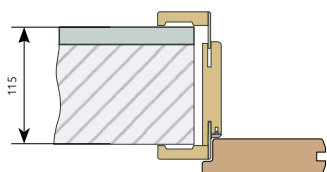
obl. zárubeň B (95-115 mm) síla stěny 115 mm záklopový límec vysunutý v rozsahu regulace 0-20 mm na své maximum.
