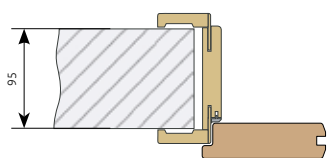
obl. zárubeň B (95-115 mm) síla stěny 95 mm zasunutý záklopový límec
